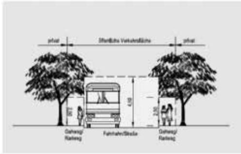
Skizze Lichtraumprofil
